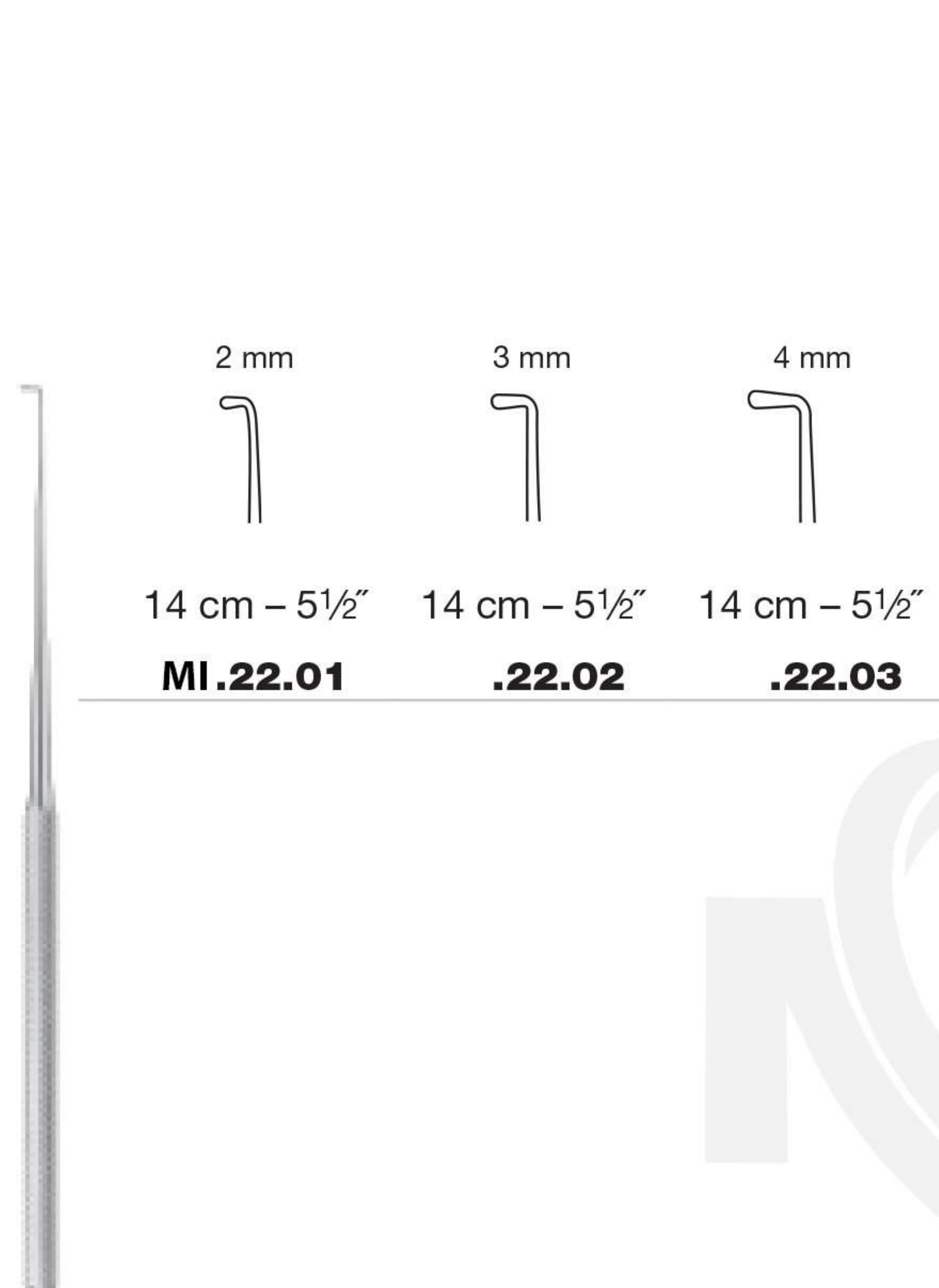
Lucae
