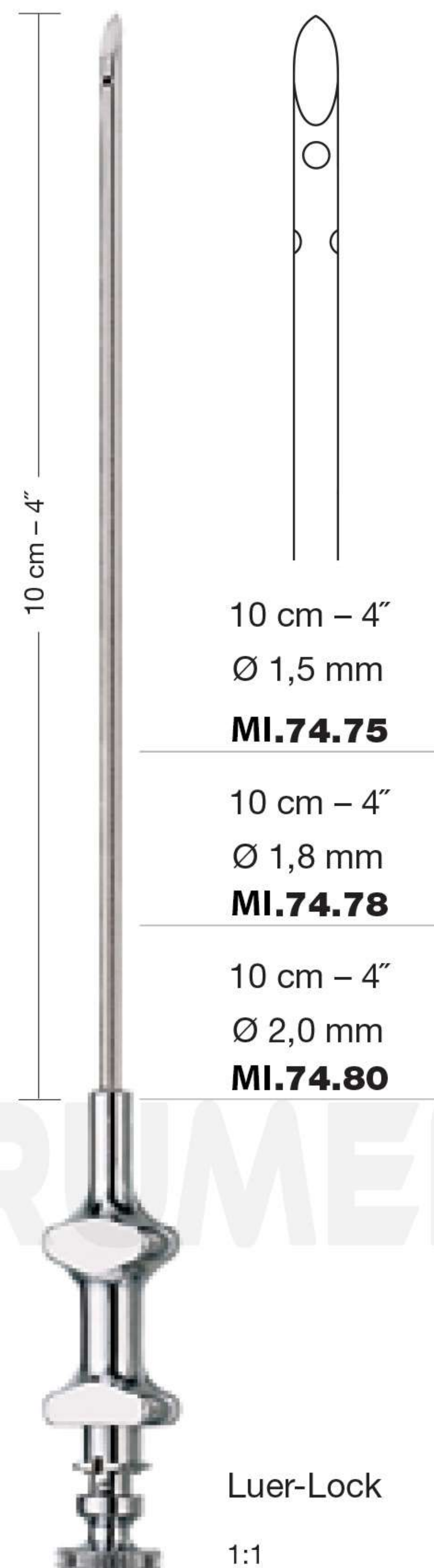
Vogel
